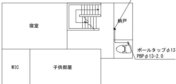
2F給水配管平面図
