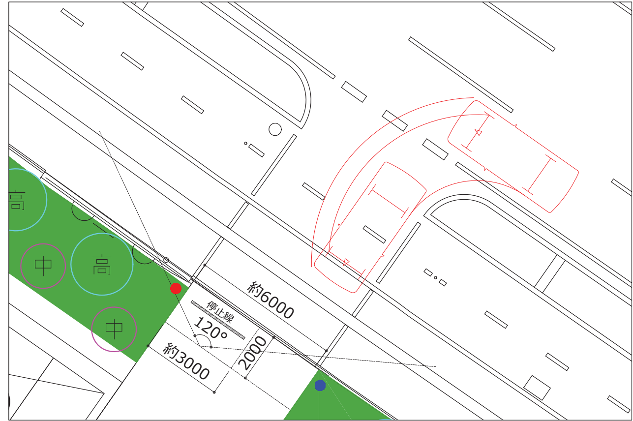
③敷地車両出入口拡大図
