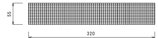
既設スリット金網 (B) 側面図
