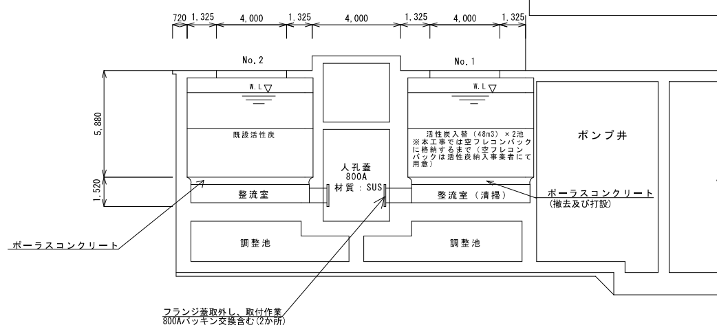
A-A断面図
