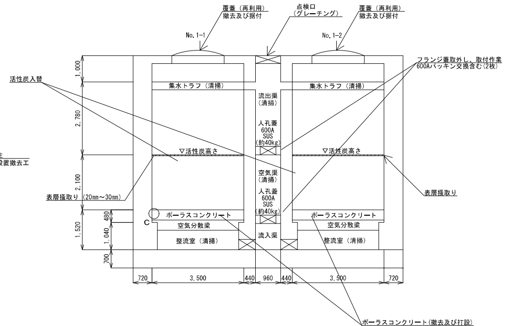
C詳細図
