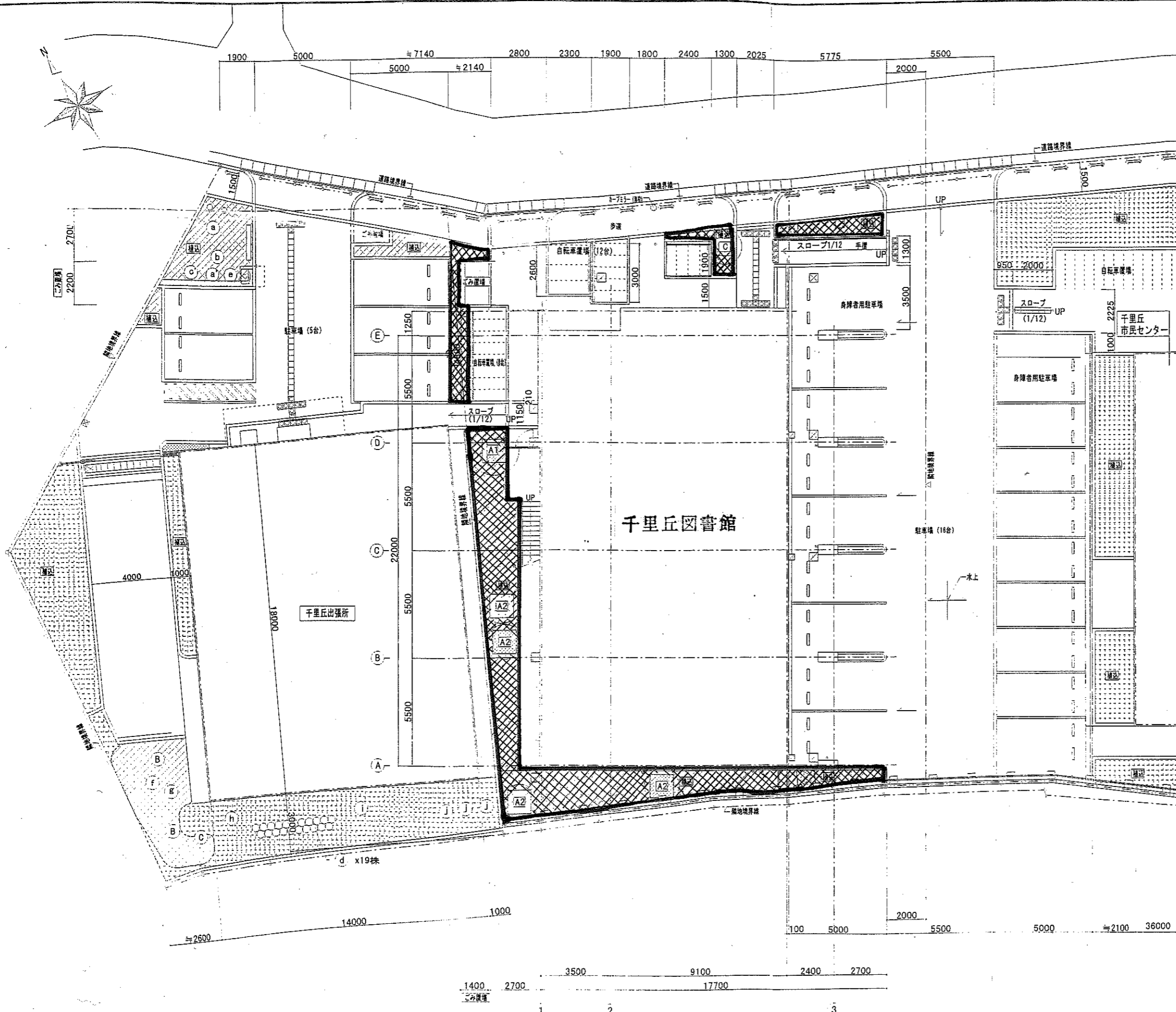
植栽計画図 1:100
