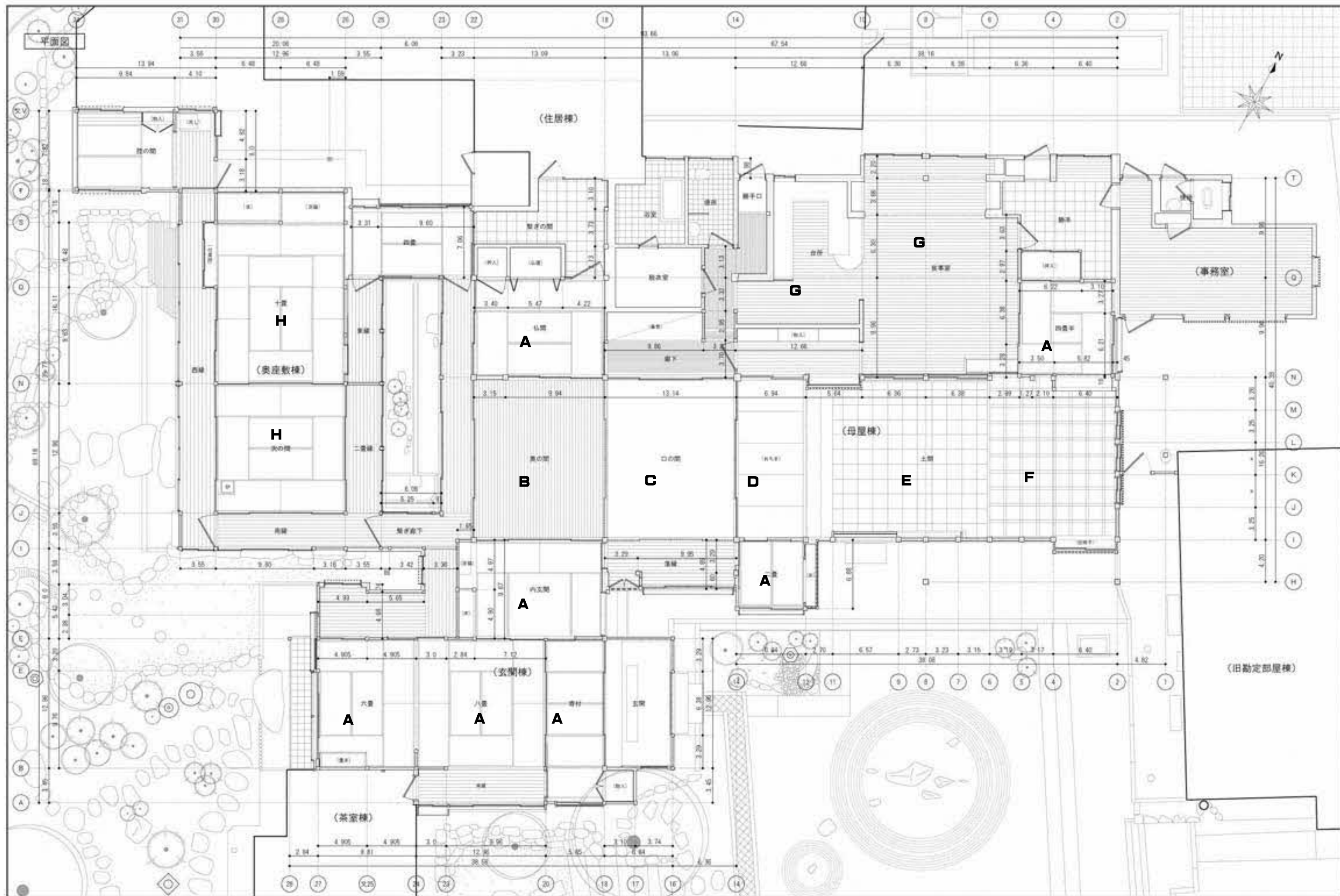
主屋平面图
