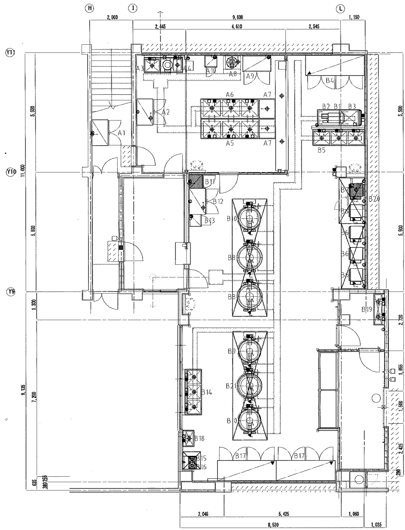
調理室 平面詳細図 縮尺 1/100
