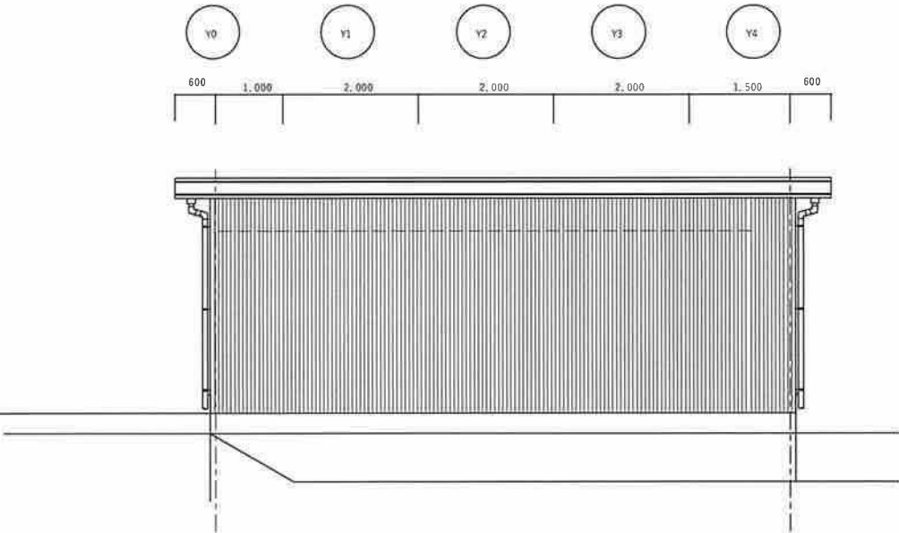
北立面図
