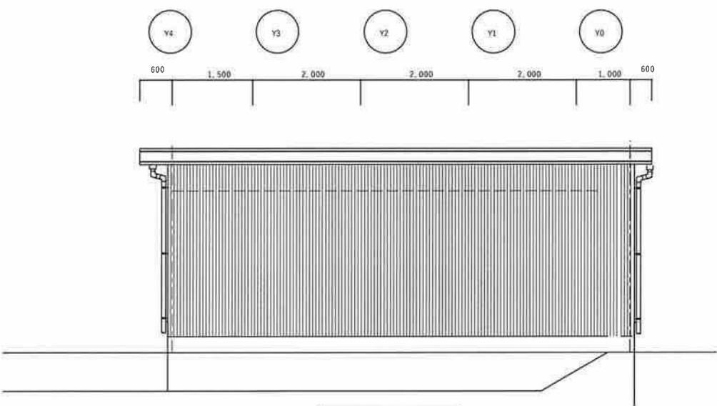
西立面図
