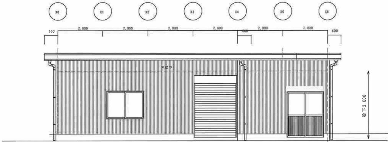
東立面図
