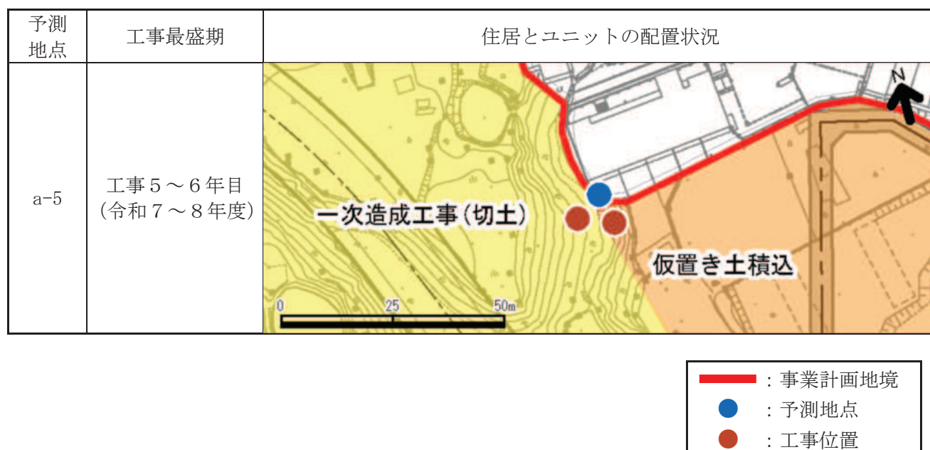
付図 5.1 住居とユニットの配置（建設機械の稼働による騒音の予測）
