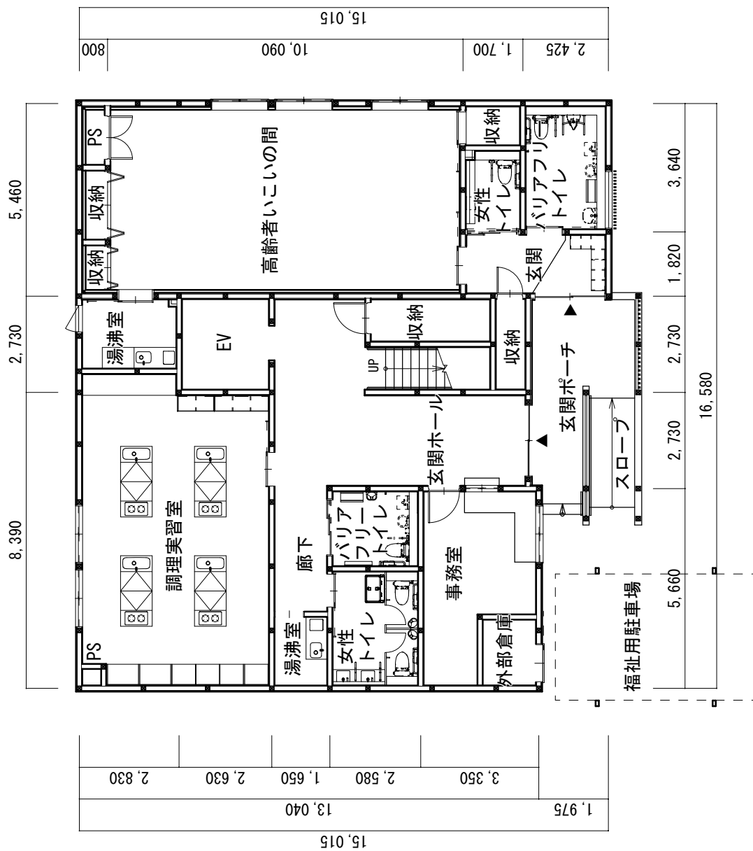
1 階平面図 1/150
