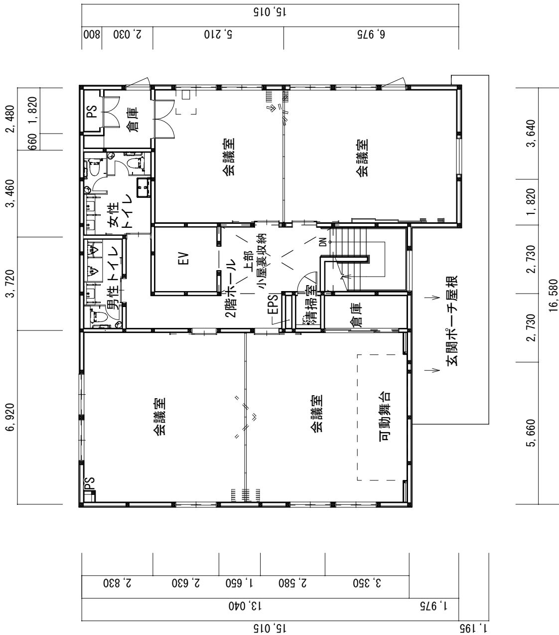
2 階平面図 1/150
