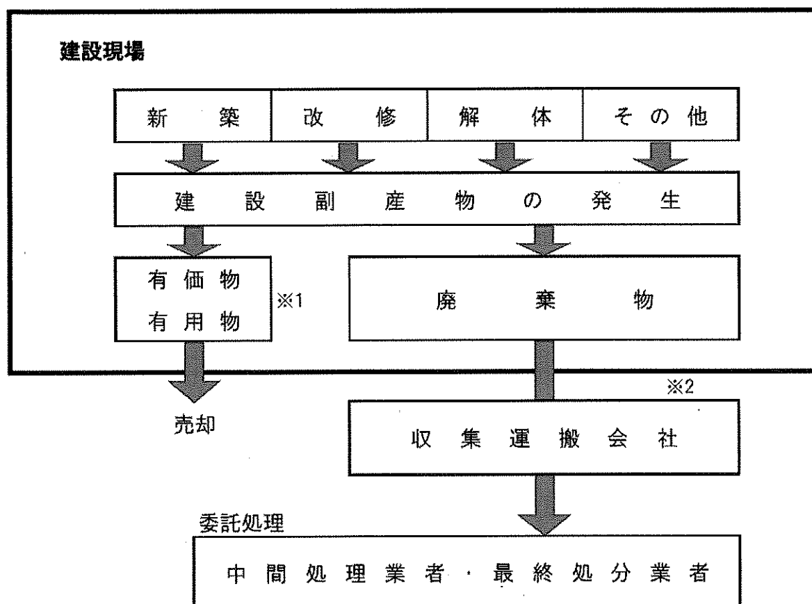
別紙(3) 産業廃棄物の一連の処理工程図
