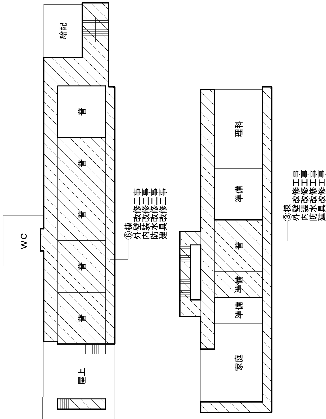
3 階平面図 1/400
