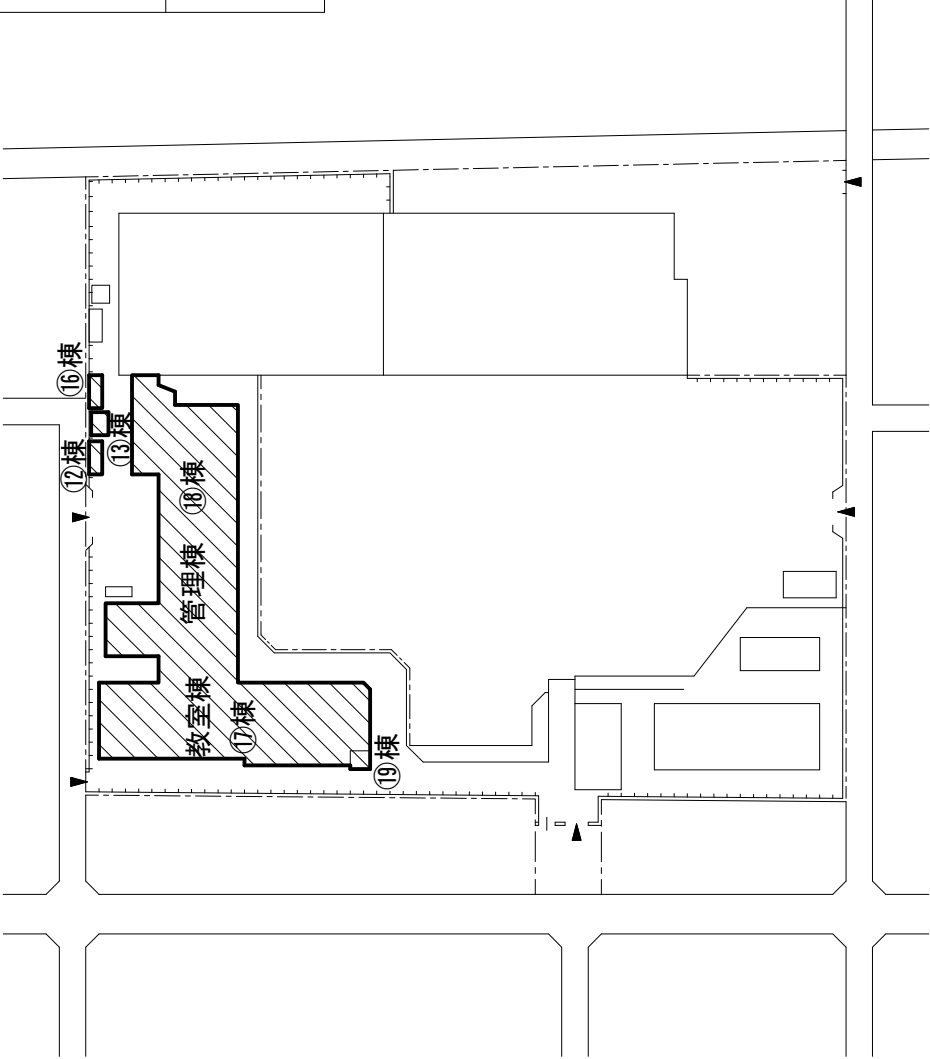
配置図 1/1200
