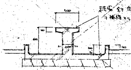
基礎詳細図 SCALE 1/50
