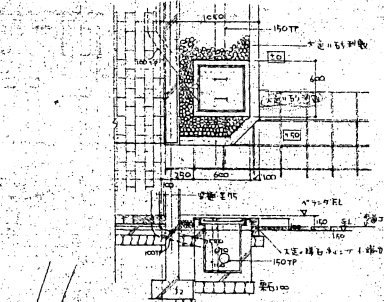
角部詳細図 1/30
