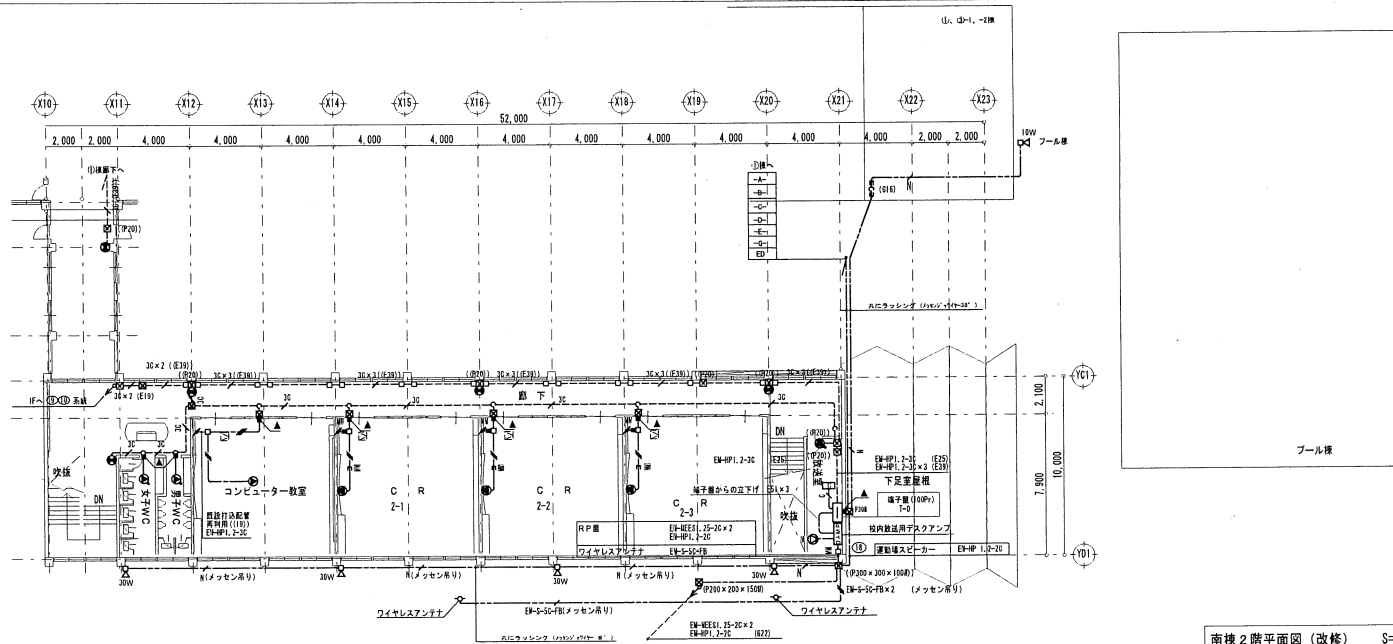
南棟 2階平面図 (改修) S=1:200
