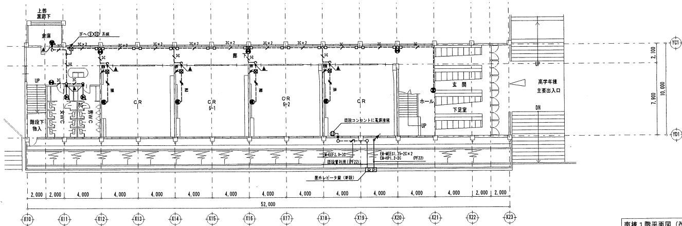
南棟 1階平面図 (改修) S=1:200
