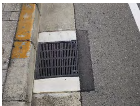
写真 5-6 グレーチング蓋の格子間隔を狭め、滑り止め加工している例（大阪市）
