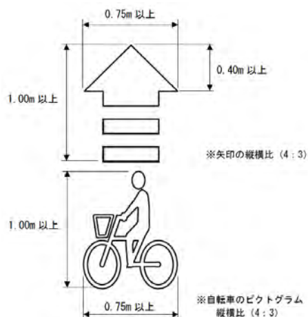
図 5-12 自転車マーク・矢印の路面表示
