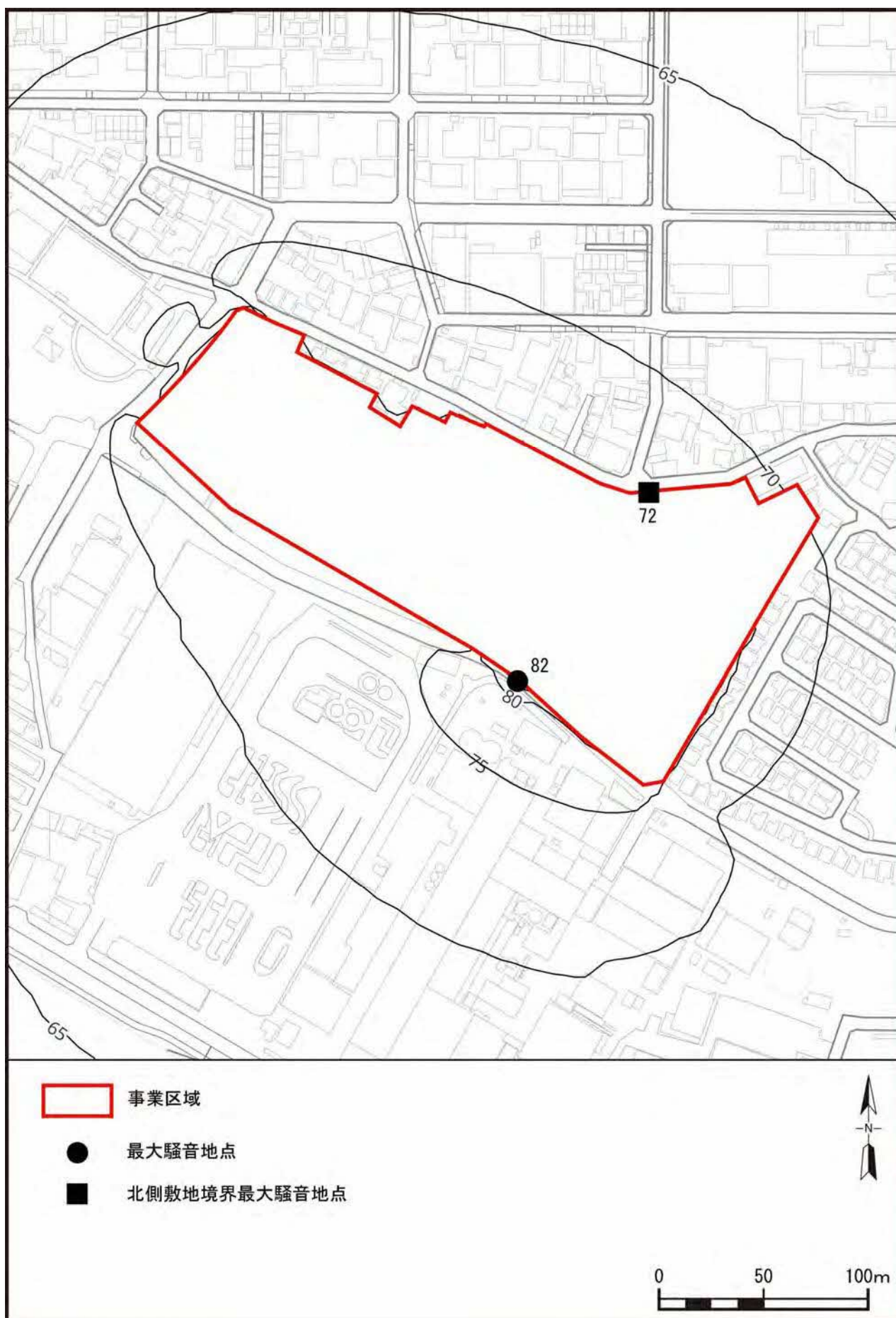
3 工区工事最盛期（着工後 21 か月目）における騒音
