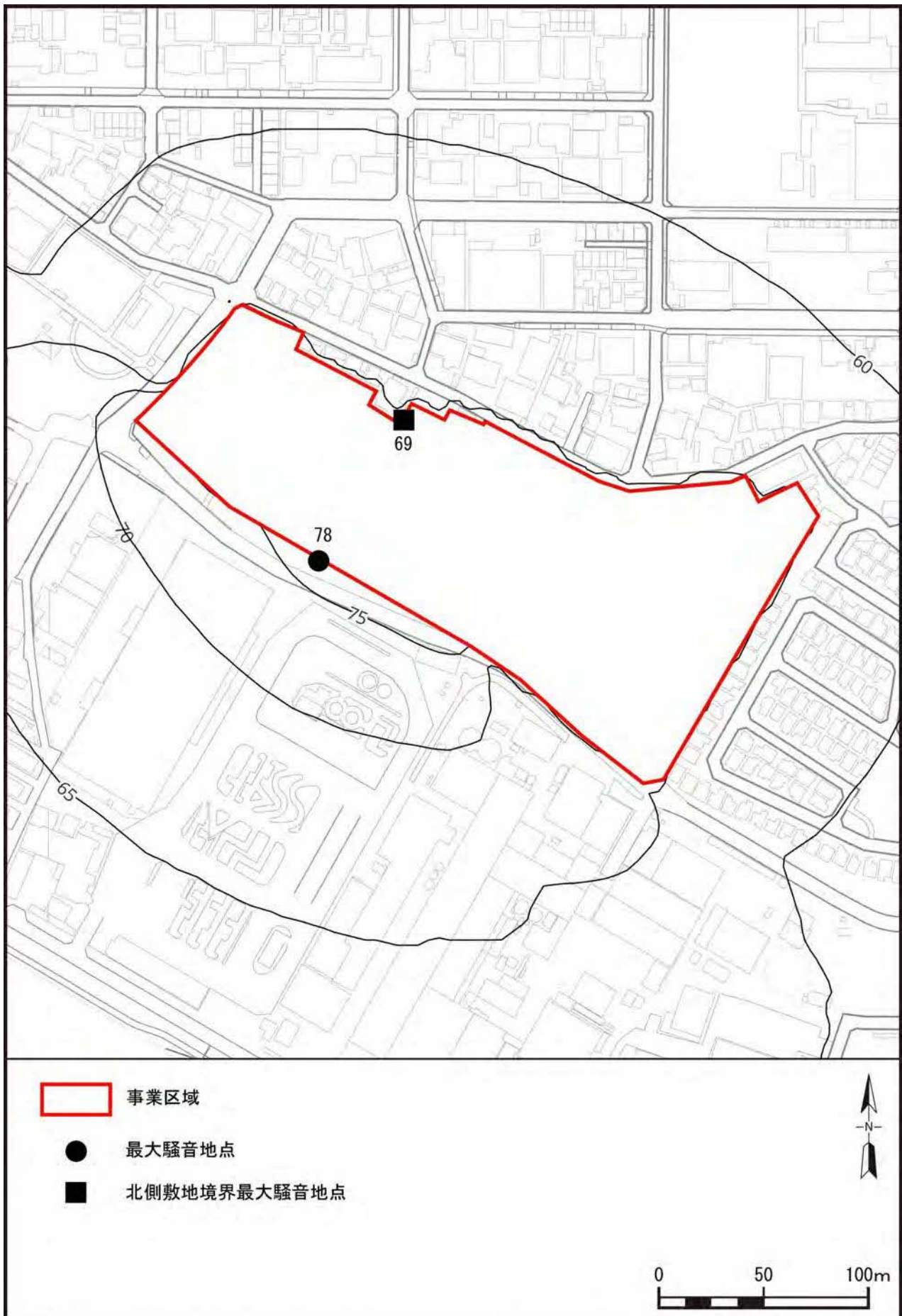
1 工区工事最盛期（着工後4か月目）における騒音
