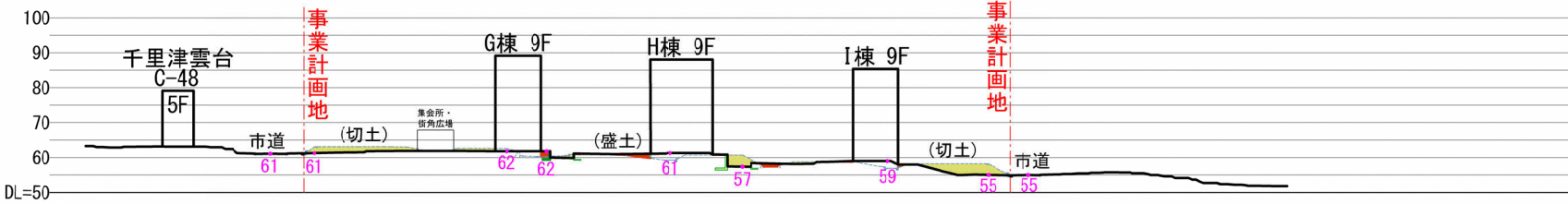
NS3－NS3断面図
