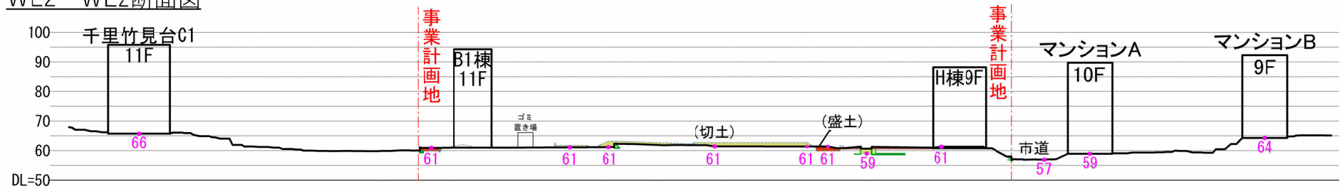
WE2－WE2断面図
