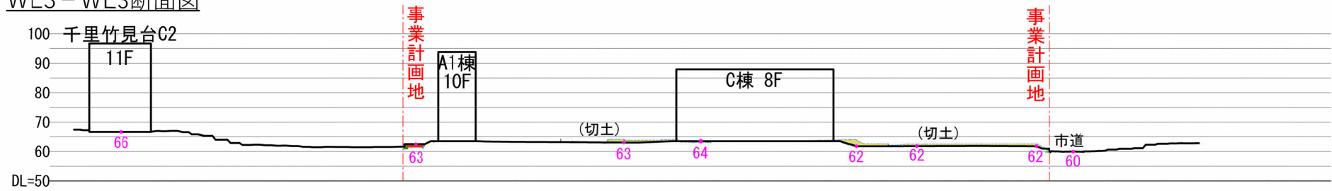
WE3－WE3断面図
