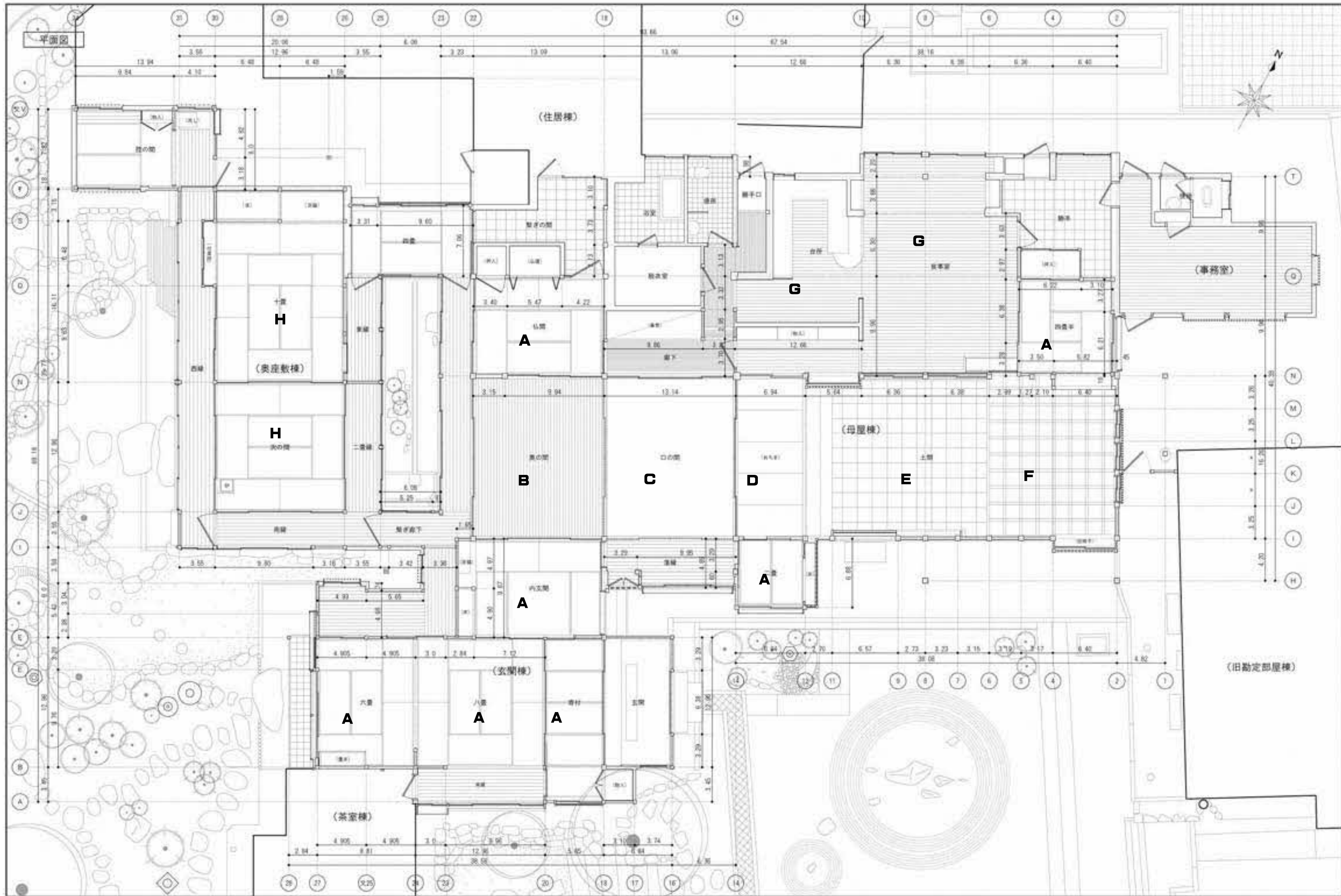
主屋平面図
