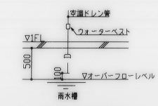
ドレン雨水槽放流部断面図
