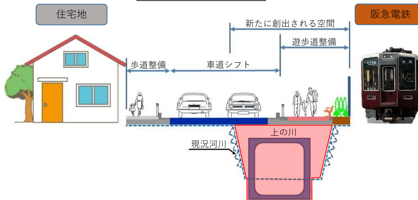
幅員構成イメージ
