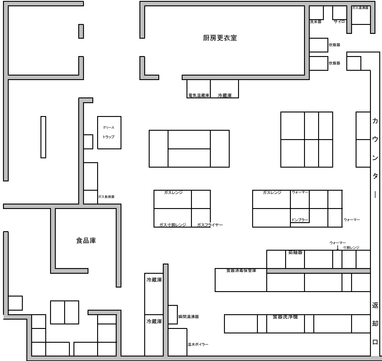
(参考) 食堂厨房設備配置図(略図)
