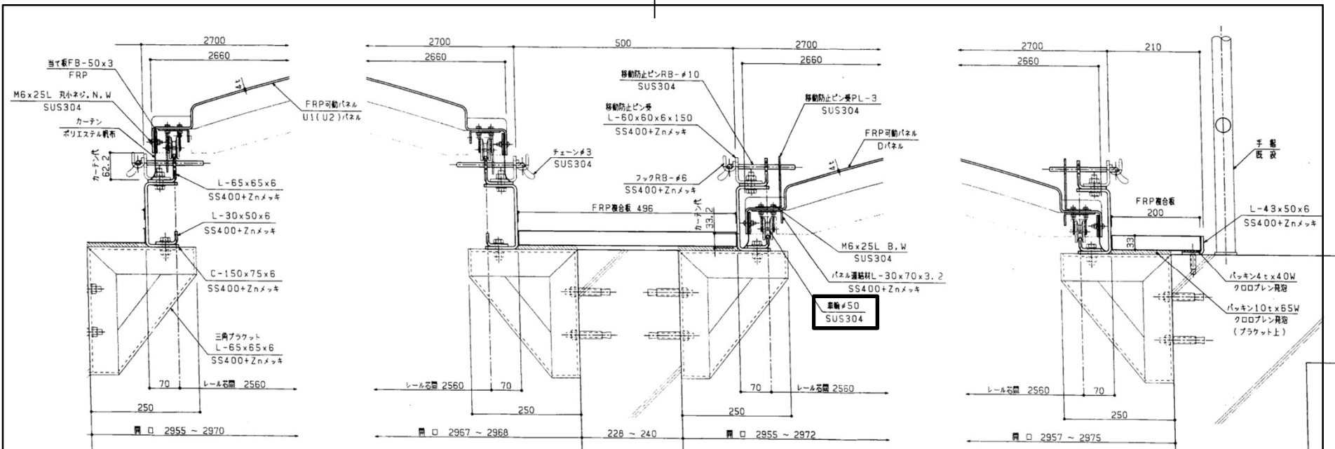
覆蓋上段取付け図
