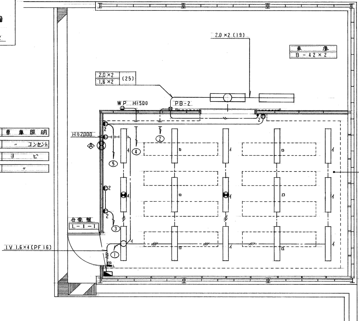
平面図
