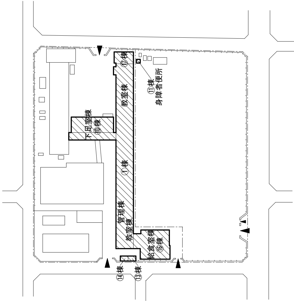
配置図 1/1200
