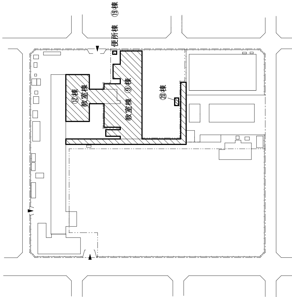
配置図 1/1200
