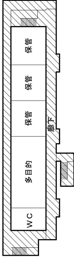
4階平面図 1/500
