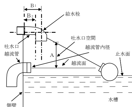
(c) 越流管（横取出し）
