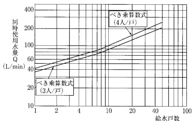
図 3 - 7 給水戸数と同時使用水量
