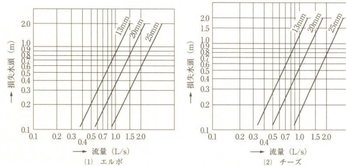
図 3 - 5 損失水頭
