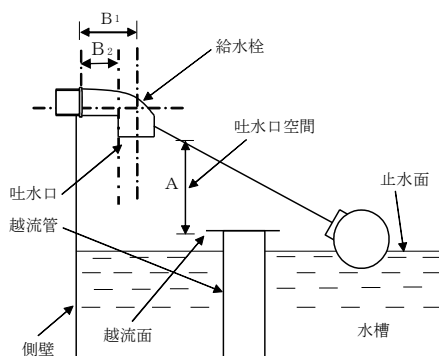
(b) 越流管（立取出し）
