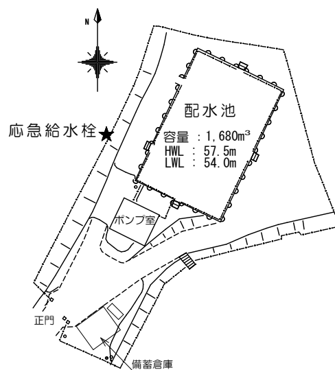
山田配水場 (S=1/1000)
