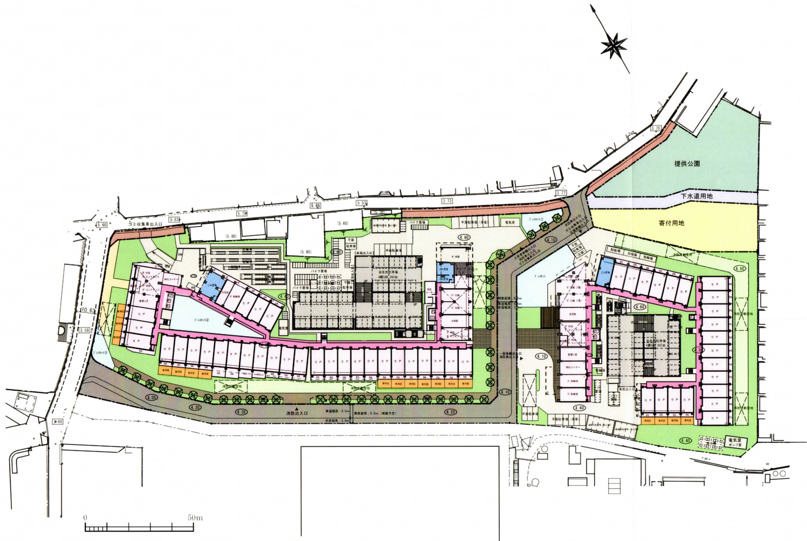
平面図（土地利用・施設計画）
