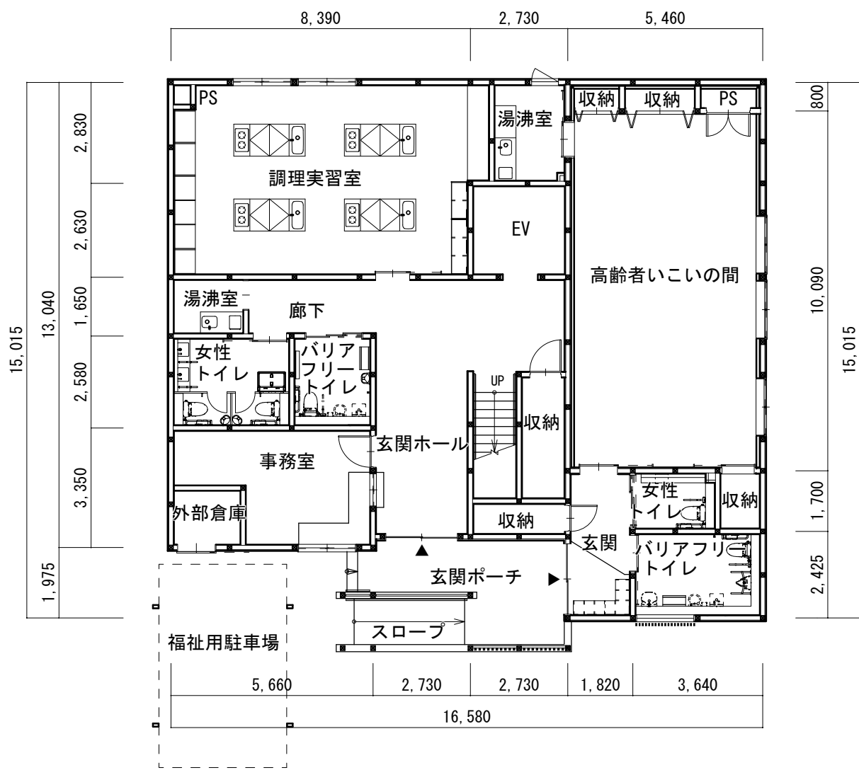
1階平面図 1/150
