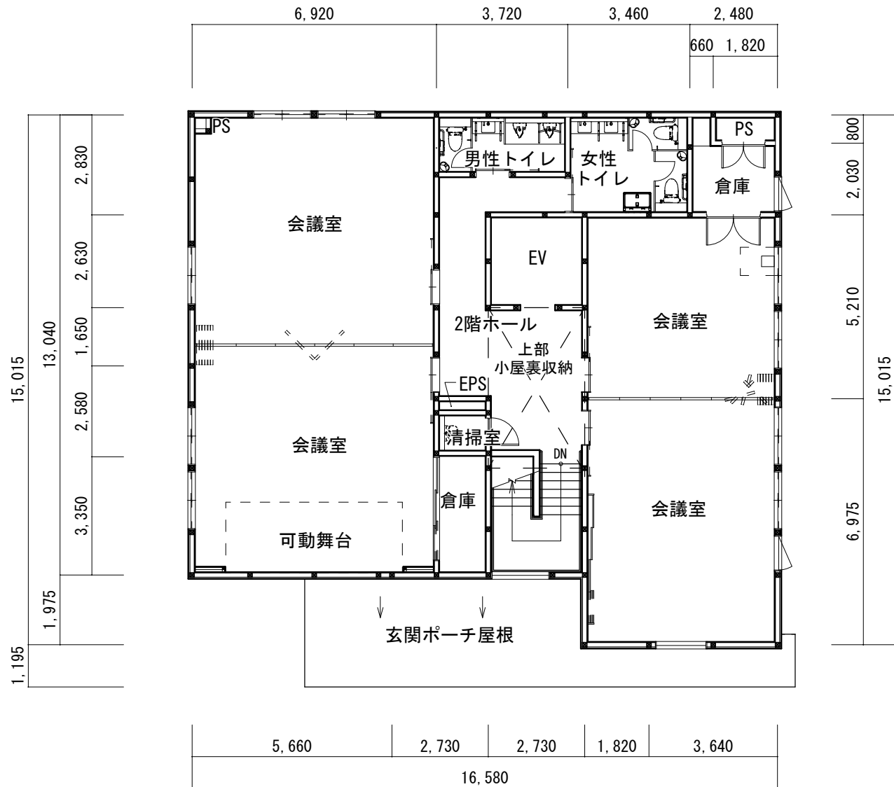
2 階平面図 1/150
