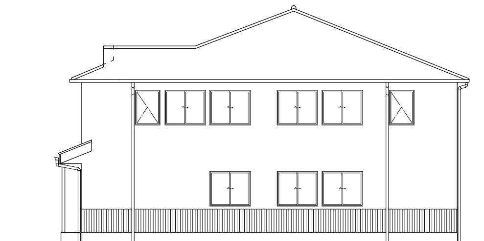
東側立面図 1/150
