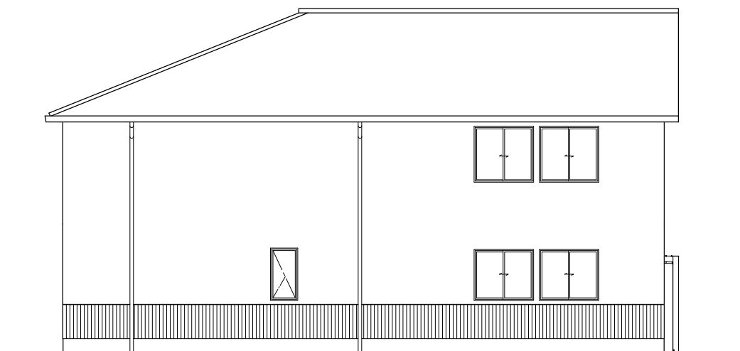
北側立面図 1/150
