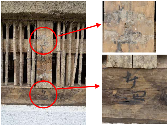
35 柱・土台墨書 柱・土台から墨書が見つかりました。ともに「廿四」(二十四)と書かれており、建設時の番付が判明しました。
