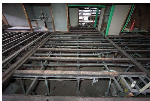
03 次の間 床板解体状況 南から見る さらに床板をめくったところです。一部の部屋の床組は近年、軽量鉄骨で補強されていました。
