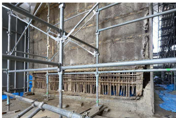
29 土壁解体状況 揚屋の準備として、足元の壁を小舞を残して解体した状況です。
