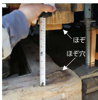
33 揚屋作業中 最終的には約 30cm 持ち上げて、土台、地覆石、柱脚部を修理できるようにしました。
