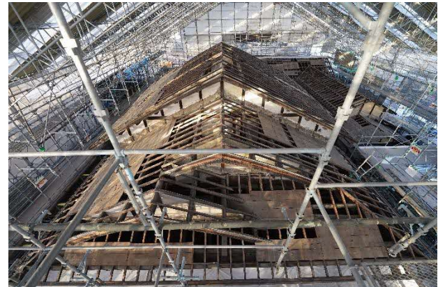
24 屋根 野地板解体 西から見る さらに野地板を一部めくったところです。なるべく材料を温存するため、解体はここまでとしました。
