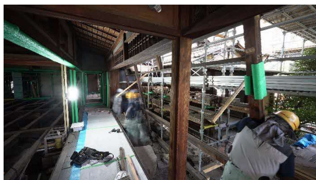
06 縁座敷 増築部分解体中 西から見る
