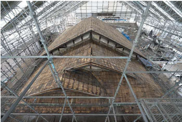
23 屋根 杉皮まで解体 西から見る 写真21の状態から、棧瓦葺、土、杉皮を解体し、野地板が見えているところです。
