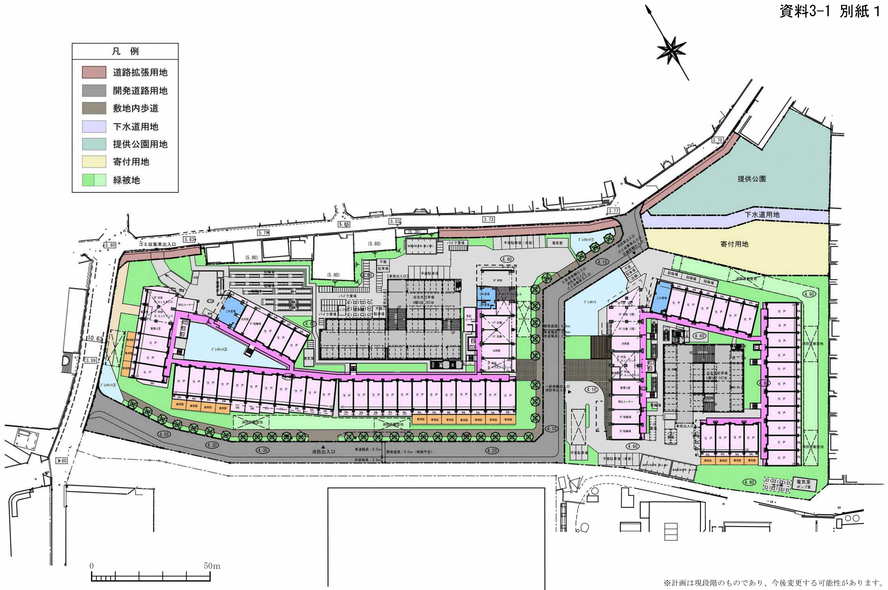
平面全体図
