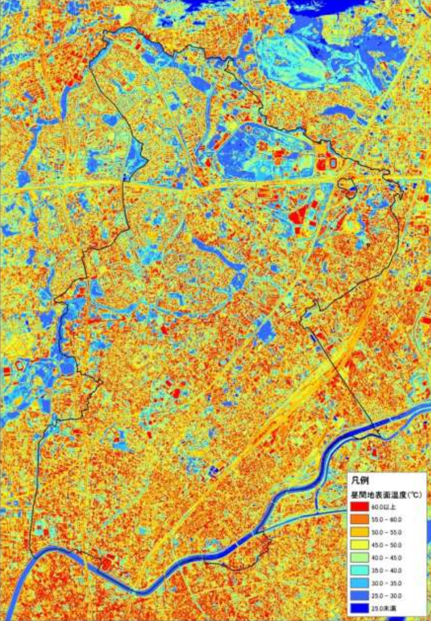
夏季昼間の地表面温度 (平成 23 年 8 月 11 日)
