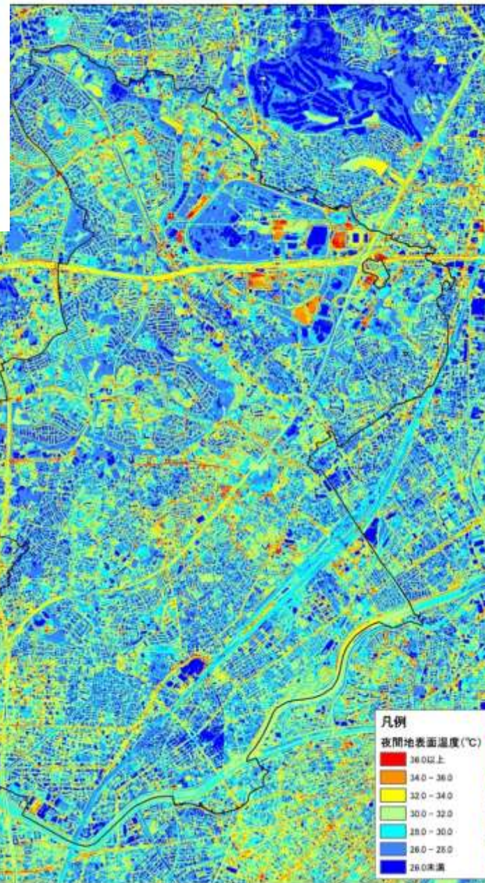
夏季夜間の地表面温度 (平成 23 年 8 月 10 日)
