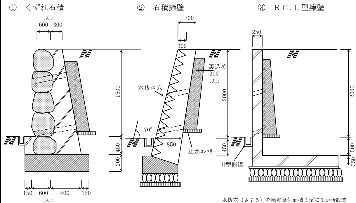
標準断面図
