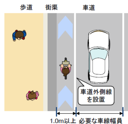
図 2-10 車道混在における車道外側線の設置
