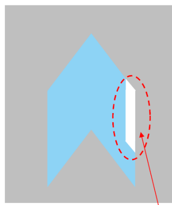
図 2-5 矢羽根型路面表示の標準仕様(案)
