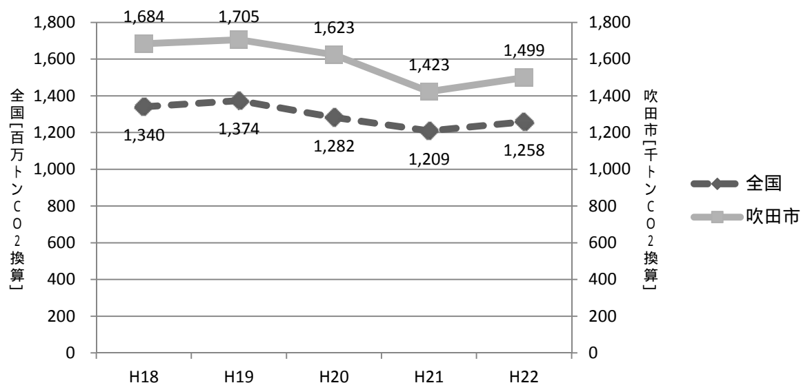
【本市及び日本の温室効果ガス排出量の推移】
