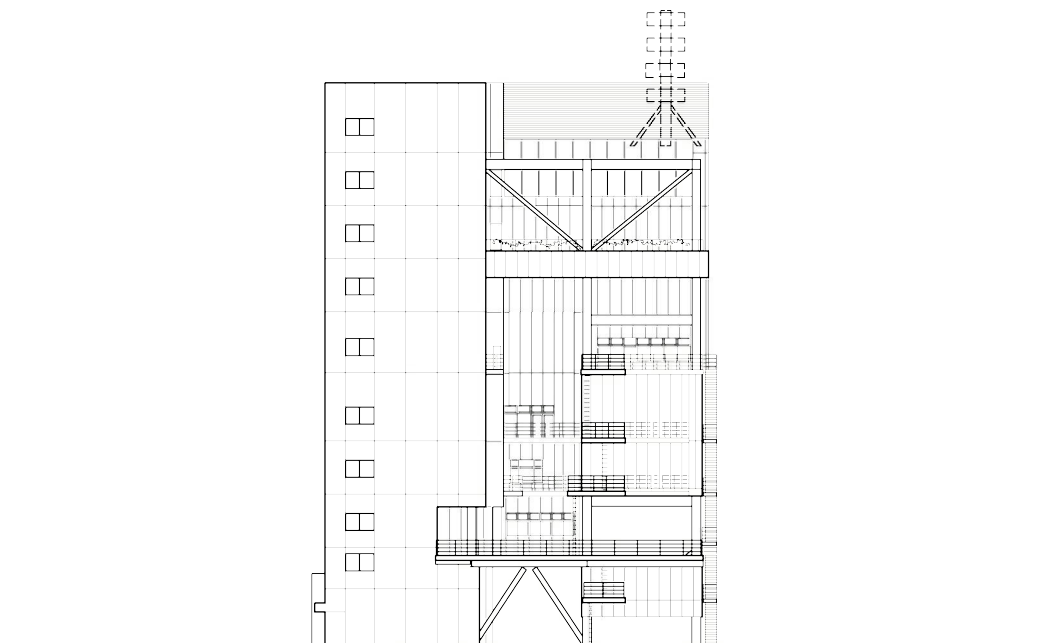
南立面図 S=1 : 600
