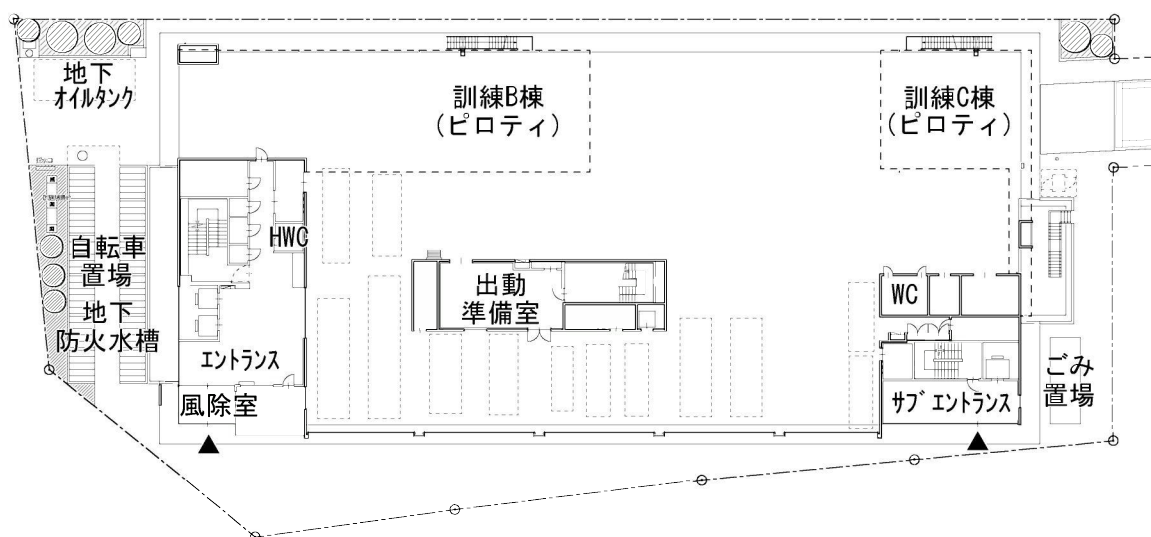
1階平面図 S=1 : 600
