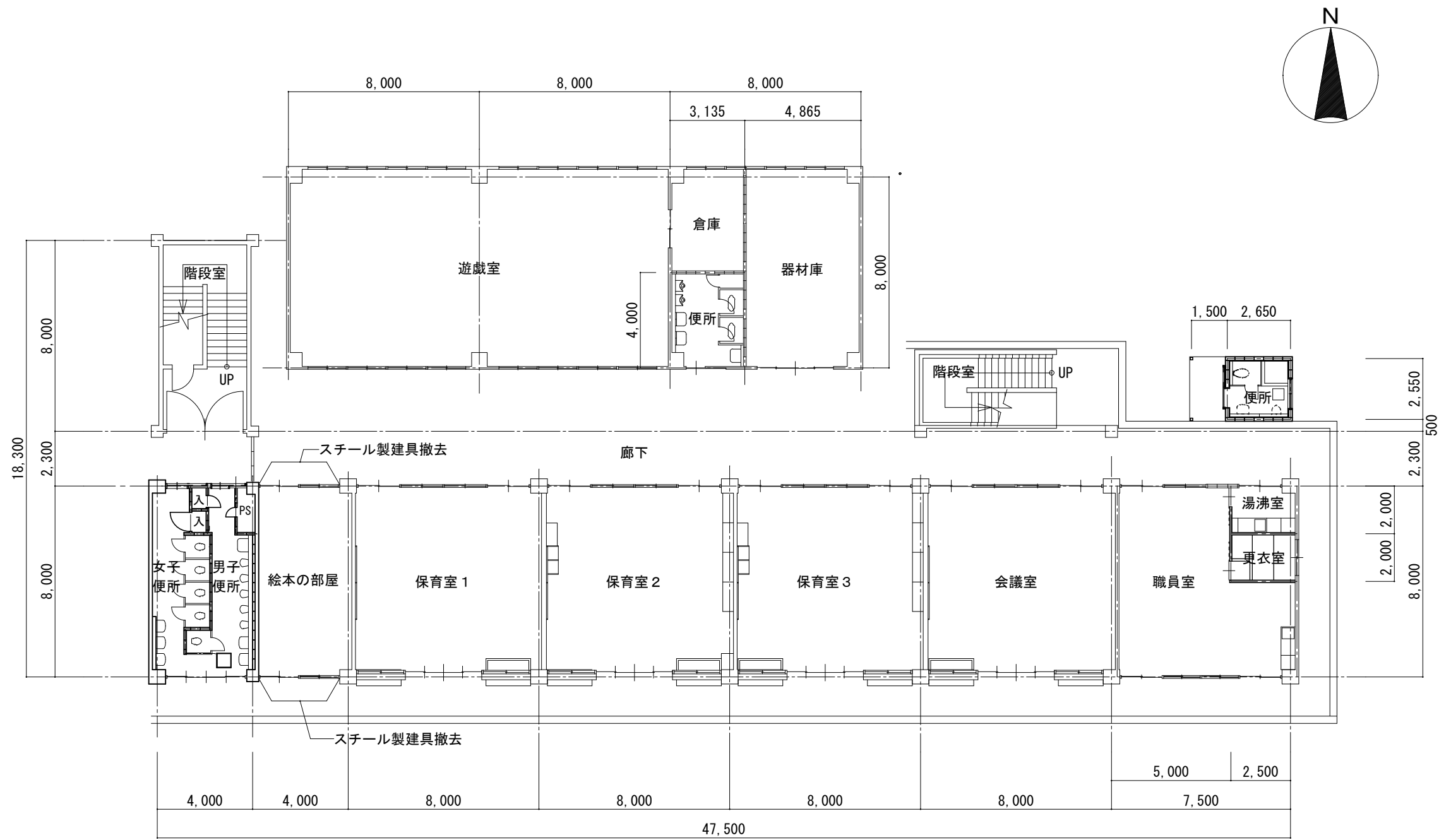
平面図 (改修前) 1/200
