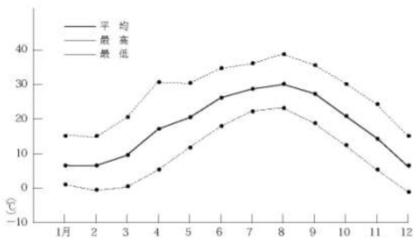
平成17年（2005年）月別気温
