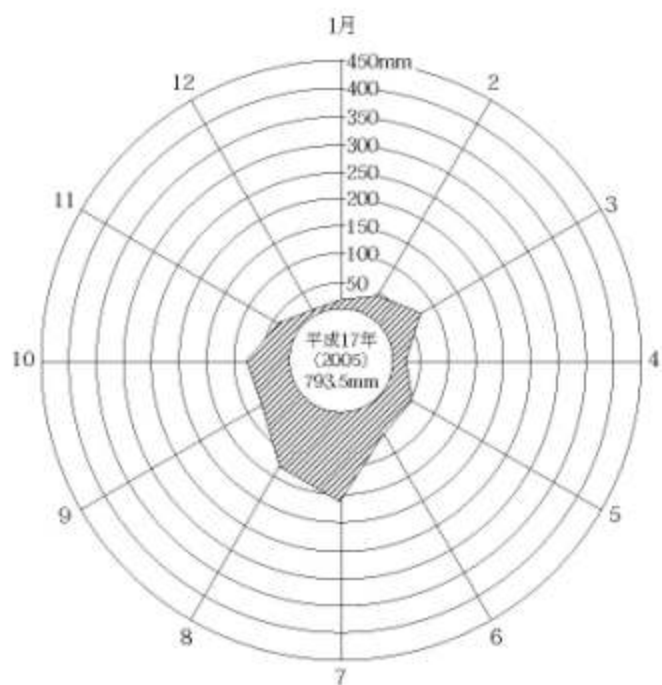
平成17年（2005年）月別降水量
