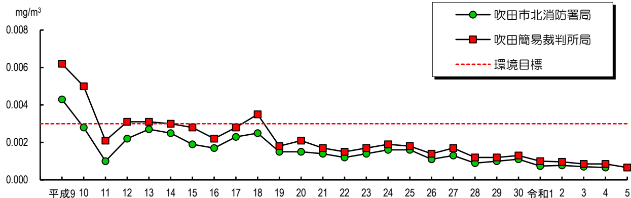
トリクロロエチレン濃度の経年変化（年平均値）
