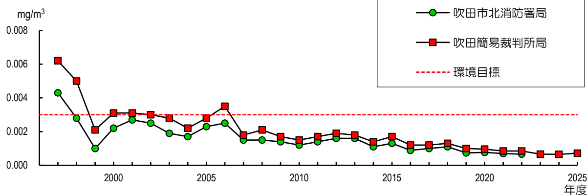
トリクロロエチレン濃度の経年変化（年平均値）
