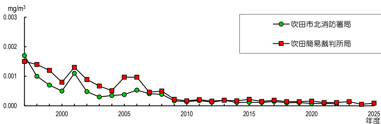
ジクロロメタン濃度の経年変化（年平均値）
