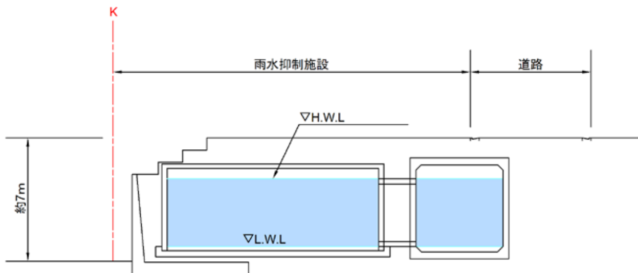
雨水流出抑制施設計画図(案)
