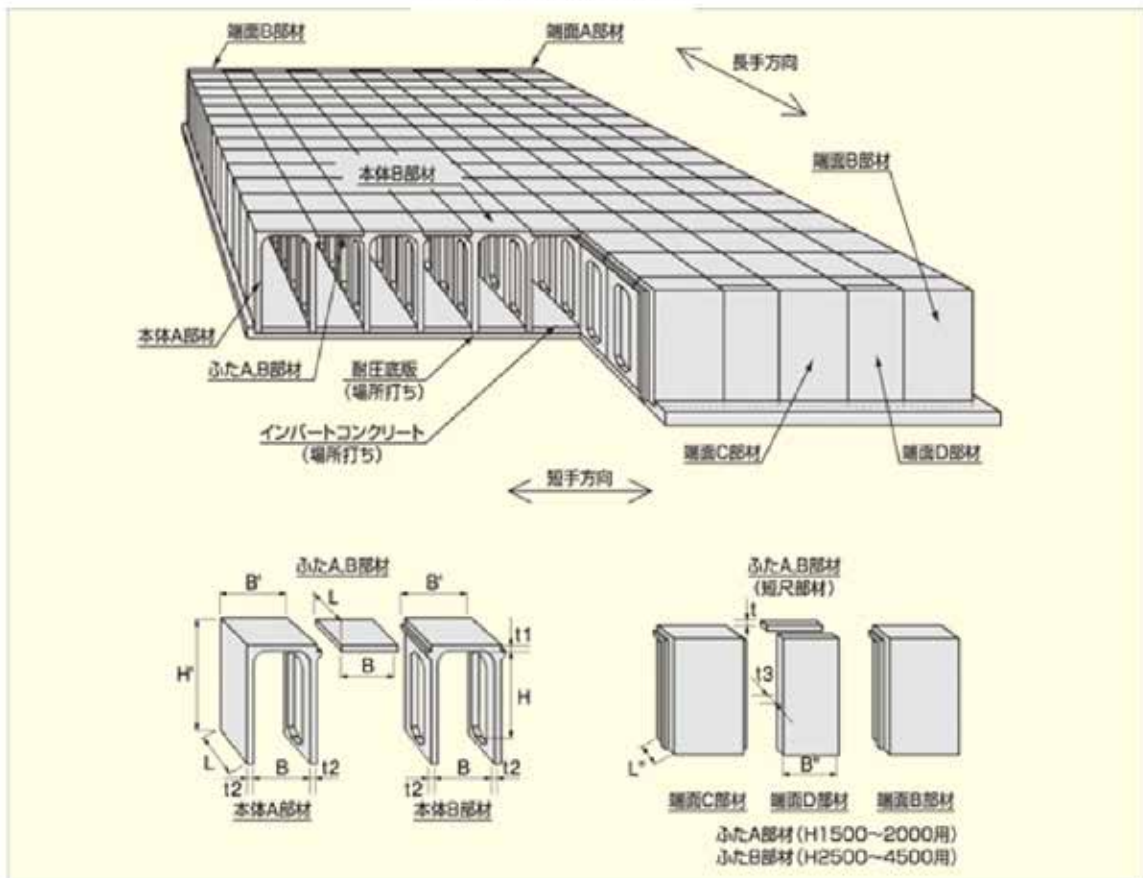
雨水流出抑制施設イメージ図
