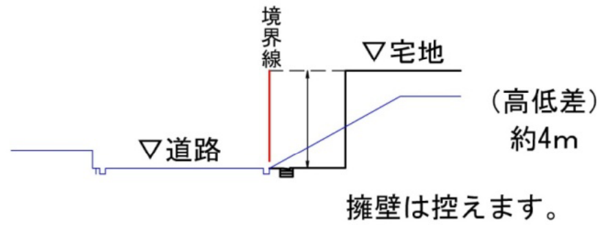
5-5' 断面図
