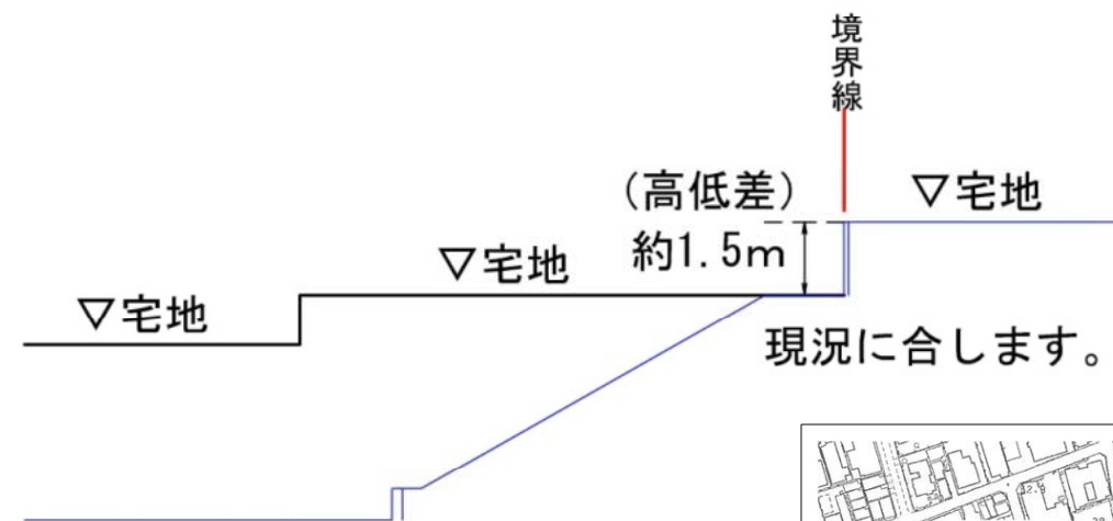
8-8' 断面図
