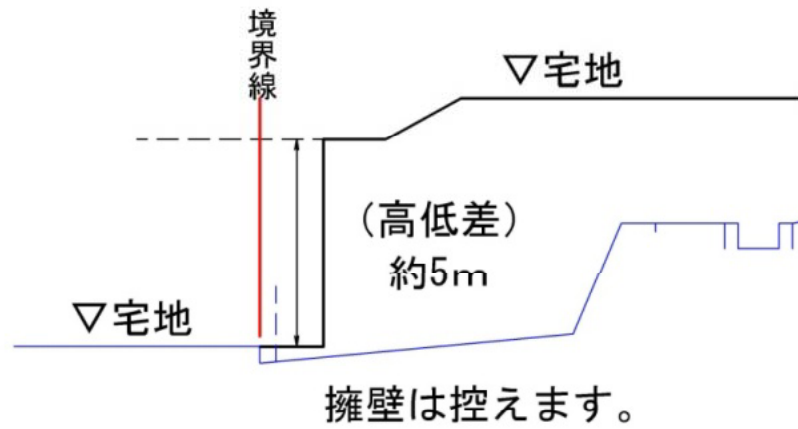
2-2' 断面図
