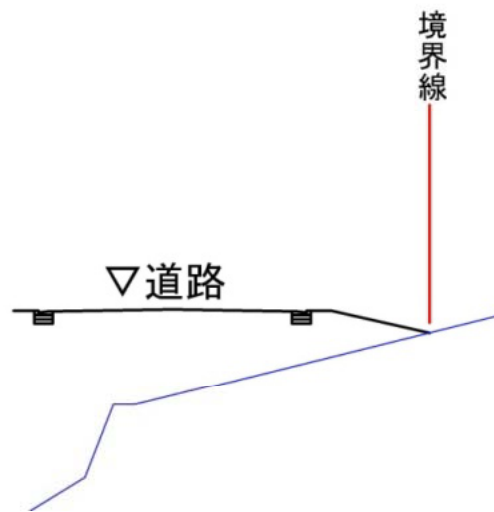
6-6' 断面図
