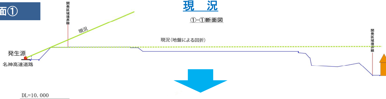
①-①断面図
