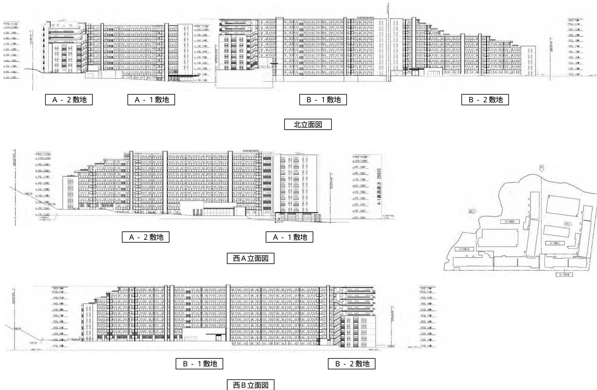
図 3-3(3) 施設立面図（集合住宅）
