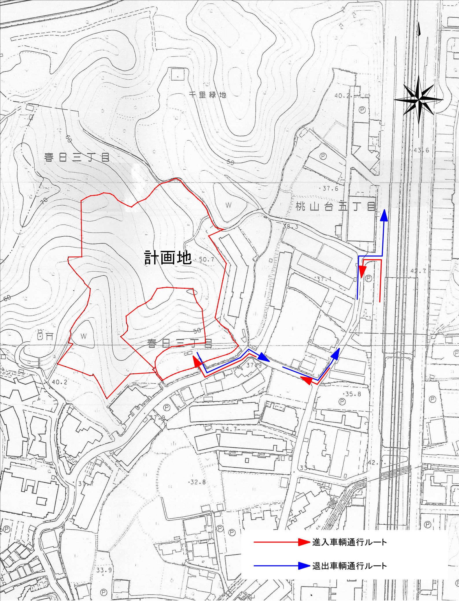
工事関連車輛通行ルート図 1/2000
