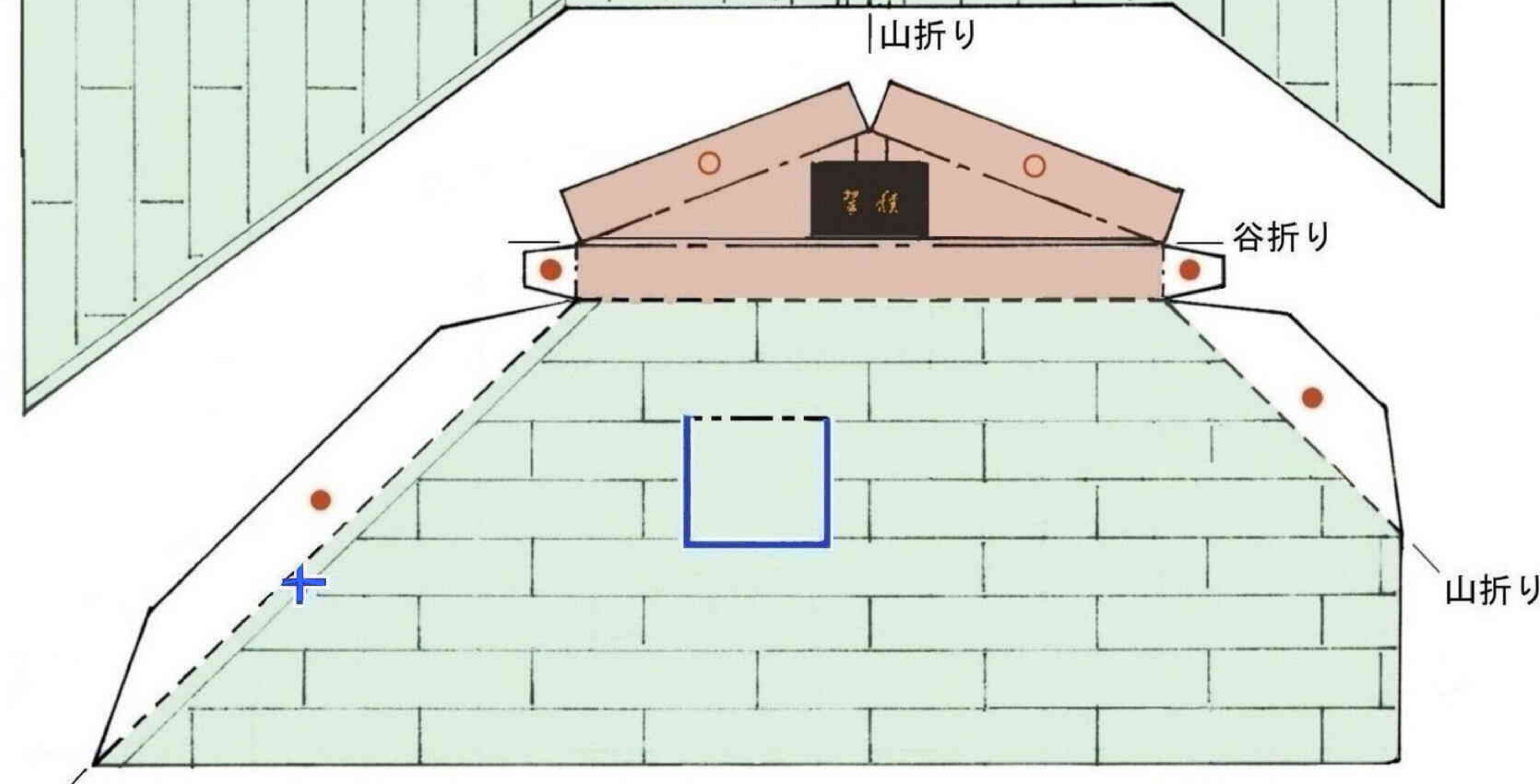
⑲南側ひさし
