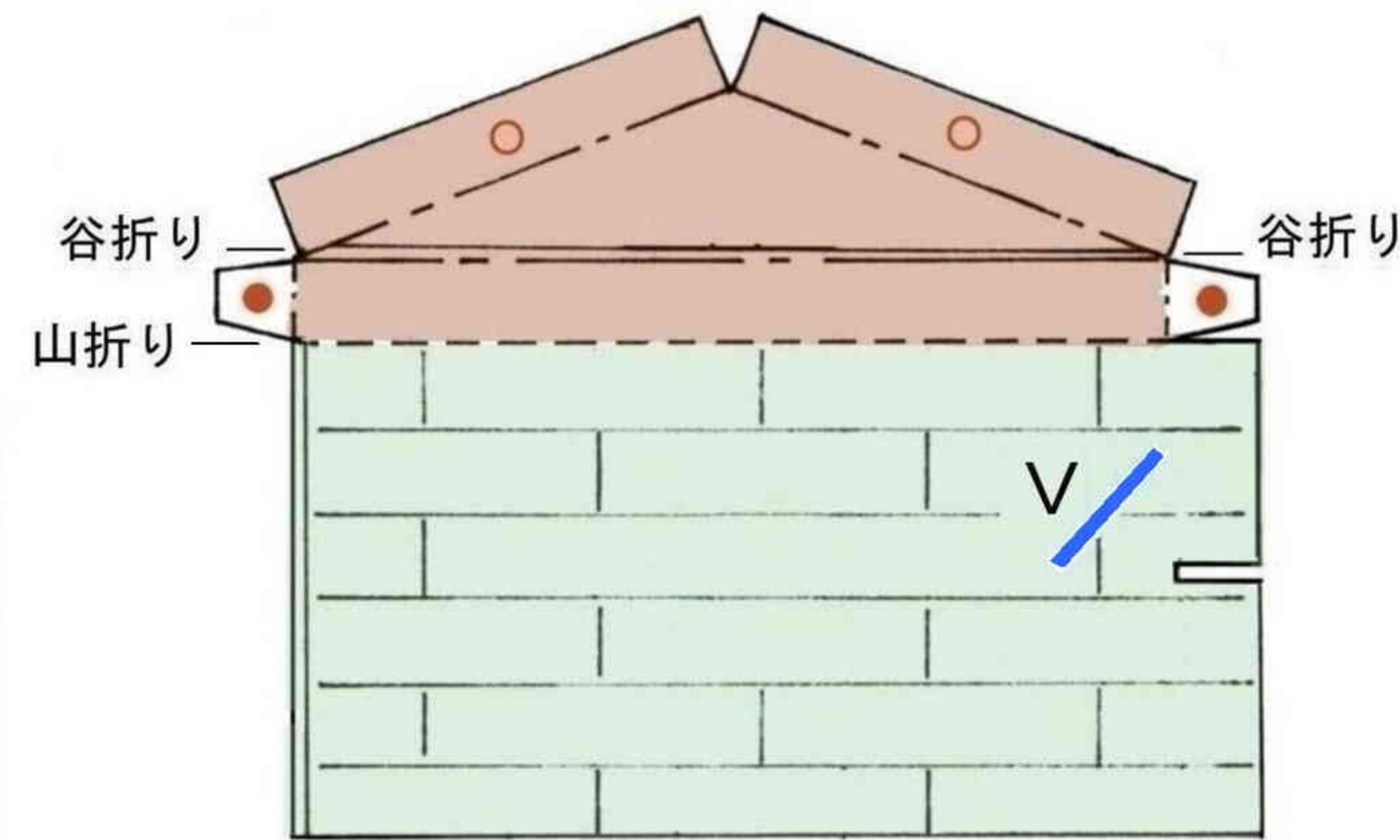
⑳北側ひさし
