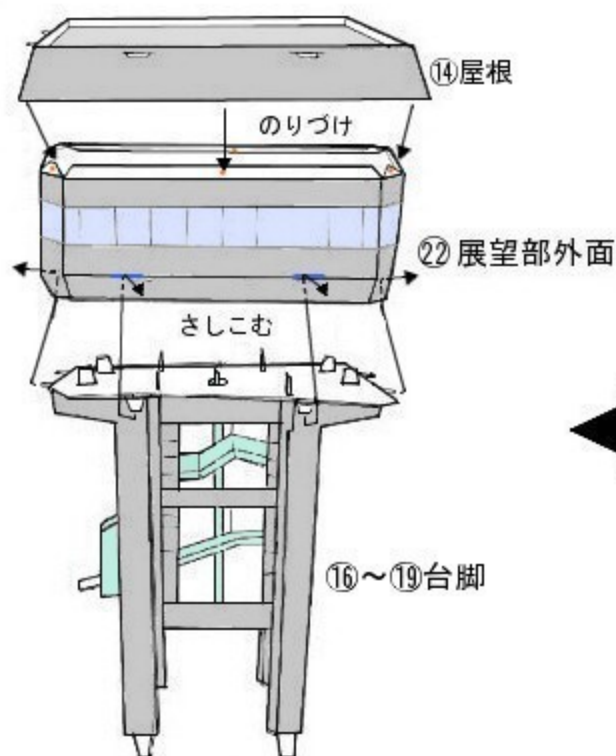
⑰～⑱台脚に㉒をさしこみ、⑭⑳をのりづけする。
