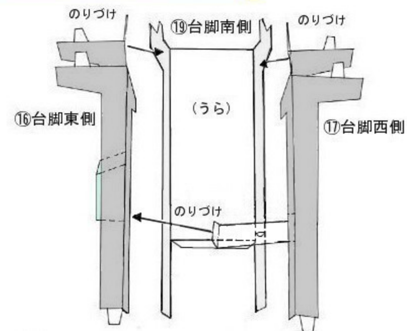
⑰に⑰⑱をのりづけする。
