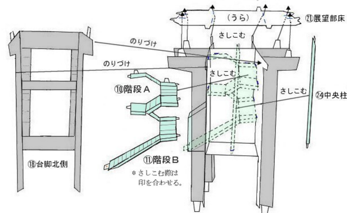
⑰⑱台脚に⑩⑪をアルファベット(a~k)に合わせて内側からさしこみ、㉔をさしこむ。その上に㉑をさしこみ、⑱をのりづけする。
