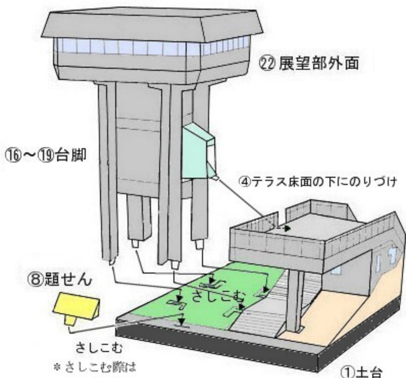
①に⑰～⑱台脚をさしこみ、⑧をさしこんで完成。
