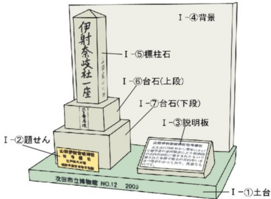
組み立て完成図
