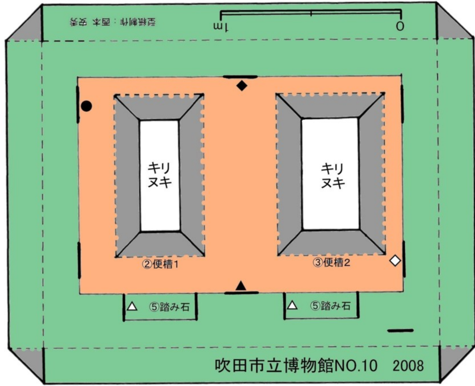
①土台
