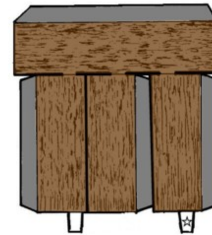
⑦ 墓室奥 柱・梁
