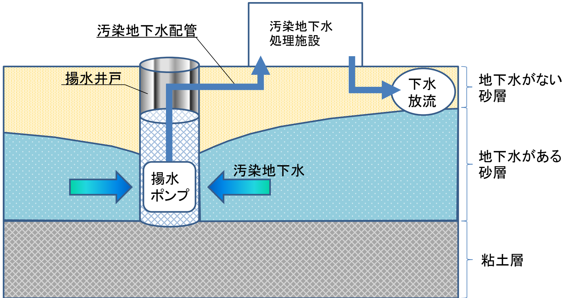
汚染拡散防止対策(揚水処理法)【概念図】
